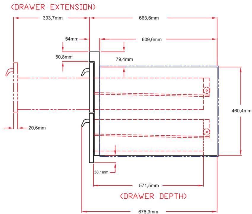
Seitenansicht
