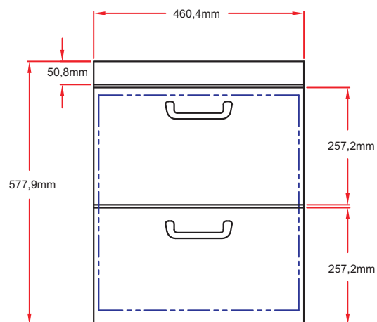
Frontansicht
