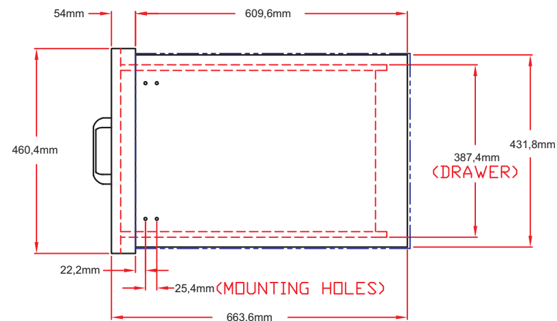
Draufsicht
