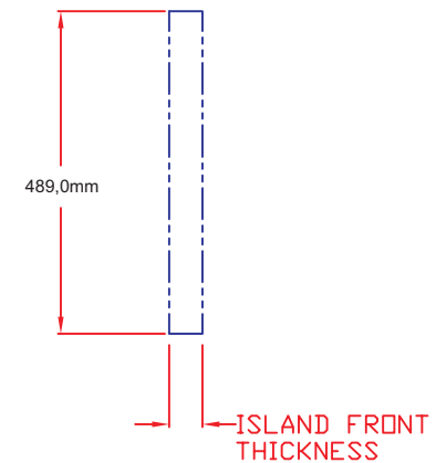
Draufsicht
